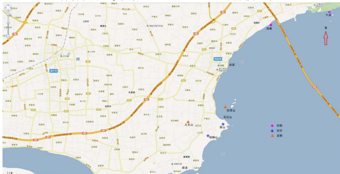
图 4：指示生物监测布点图
