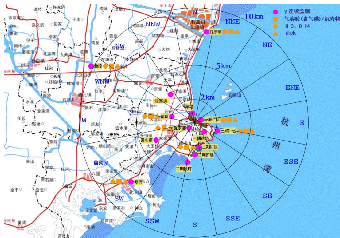
图 1: 空气样品采样点和 \gamma 连续监测点布置图
