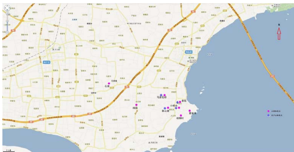
图3：陆地表层土、农产品(叶菜、萝卜、稻米)采样分布图
